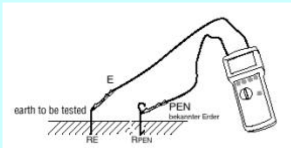
两线法测接地电阻
