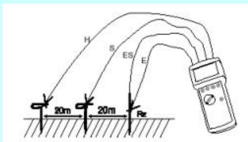
四线法测接地电阻
