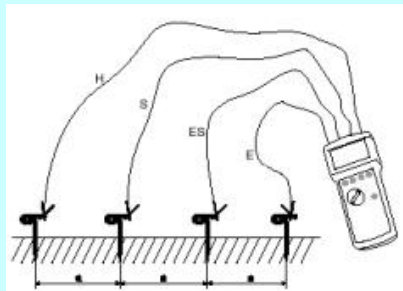
四线法测土壤电阻率
