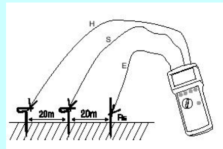
三线法测接地电阻
